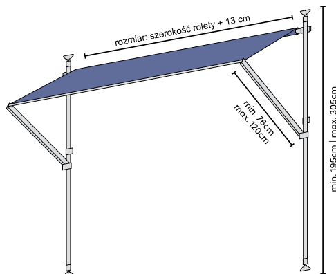
RAMA REGULOWANA FLEX FRAME® DO MARKIZY BALKONOWEJ
