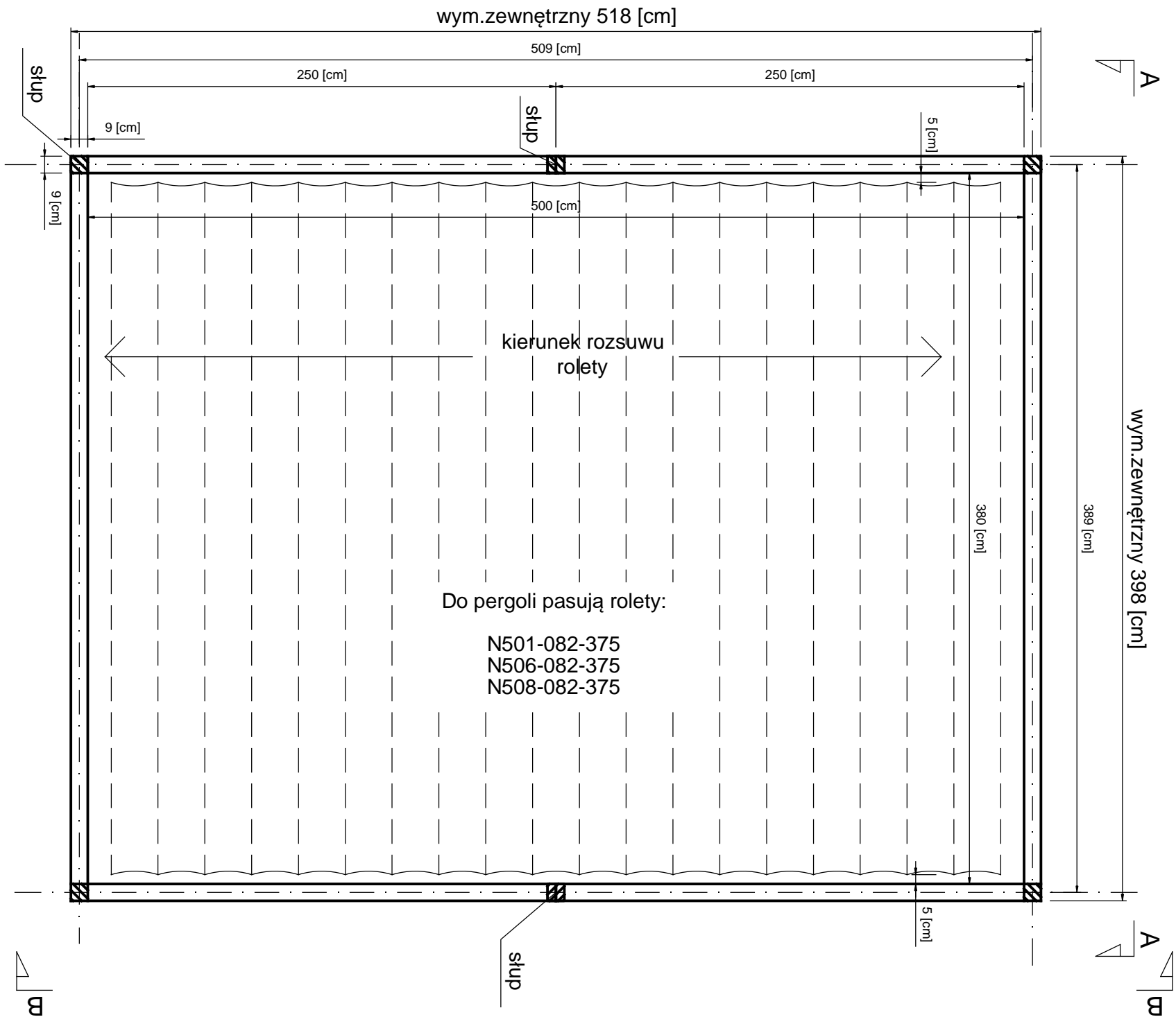
PW 370-500 rzut z góry
